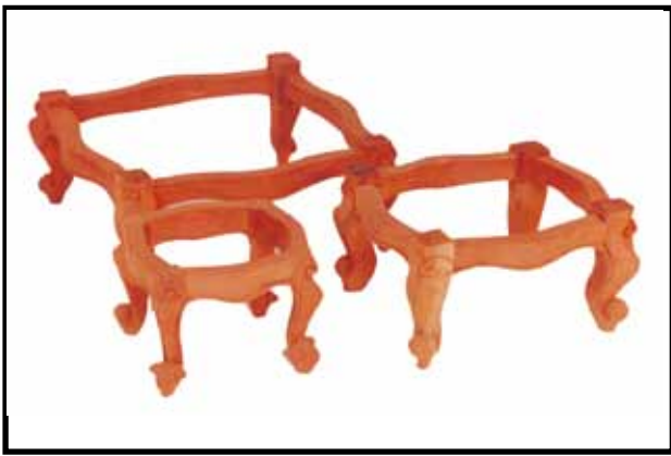
FL 011, 012 & 013 Serpentine Footstools Small - H. 14 W. 32 D. 25 Medium - H. 14 W. 41 D. 36 Large - H. 14 W. 50 D. 44
